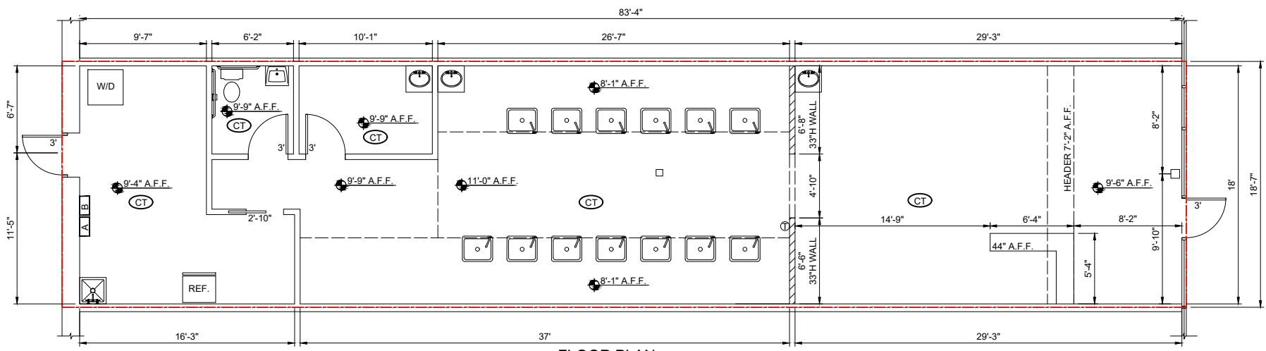
FLOOR PLAN N.T.S.
