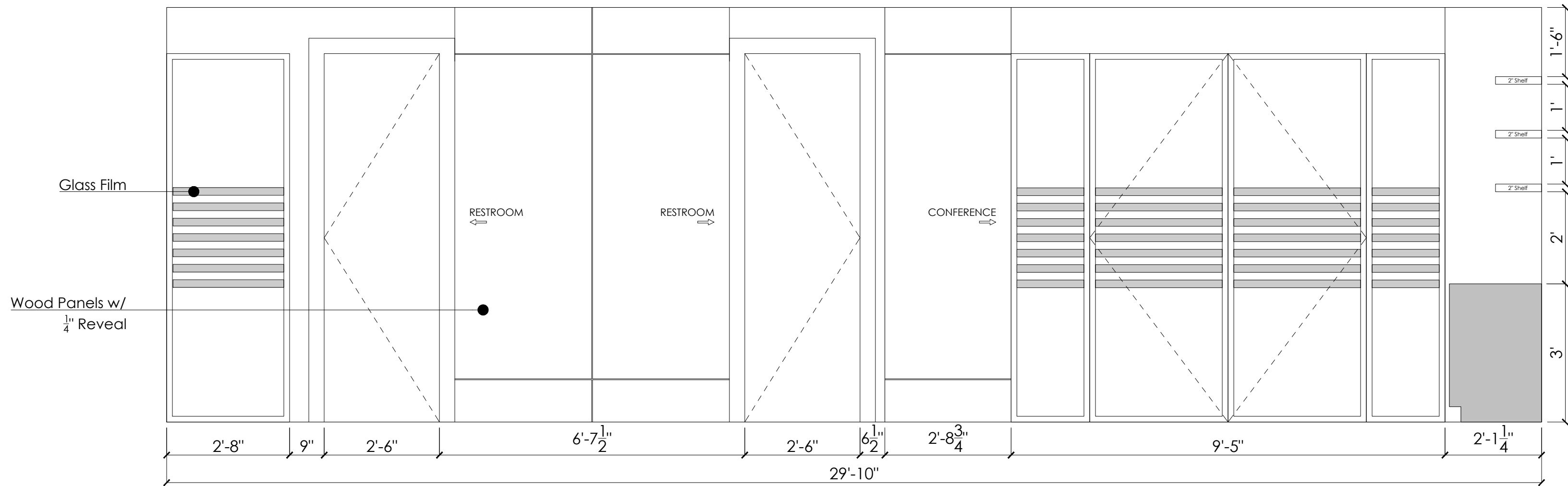
3 ELEVATION C Scale: 1/4" = 1'-0"
