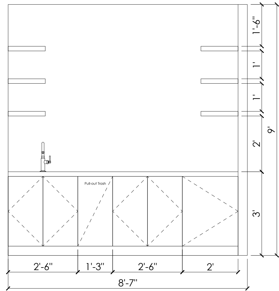
2 ELEVATION A Scale: 1/4" = 1'-0"
