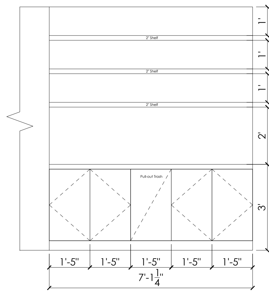
5 ELEVATION E Scale: 1/4" = 1'-0"
