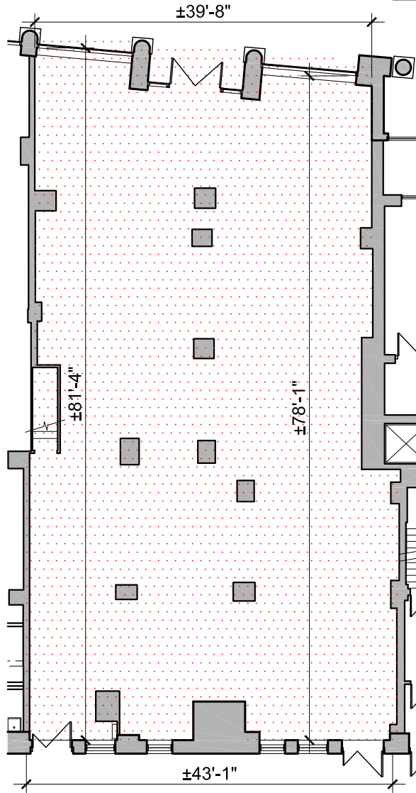
PLAN DU REZ-DE-CHAUSSÉE
