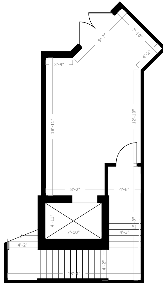
First Floor | Scale: 1/8" = 1'-0" (1=96)
