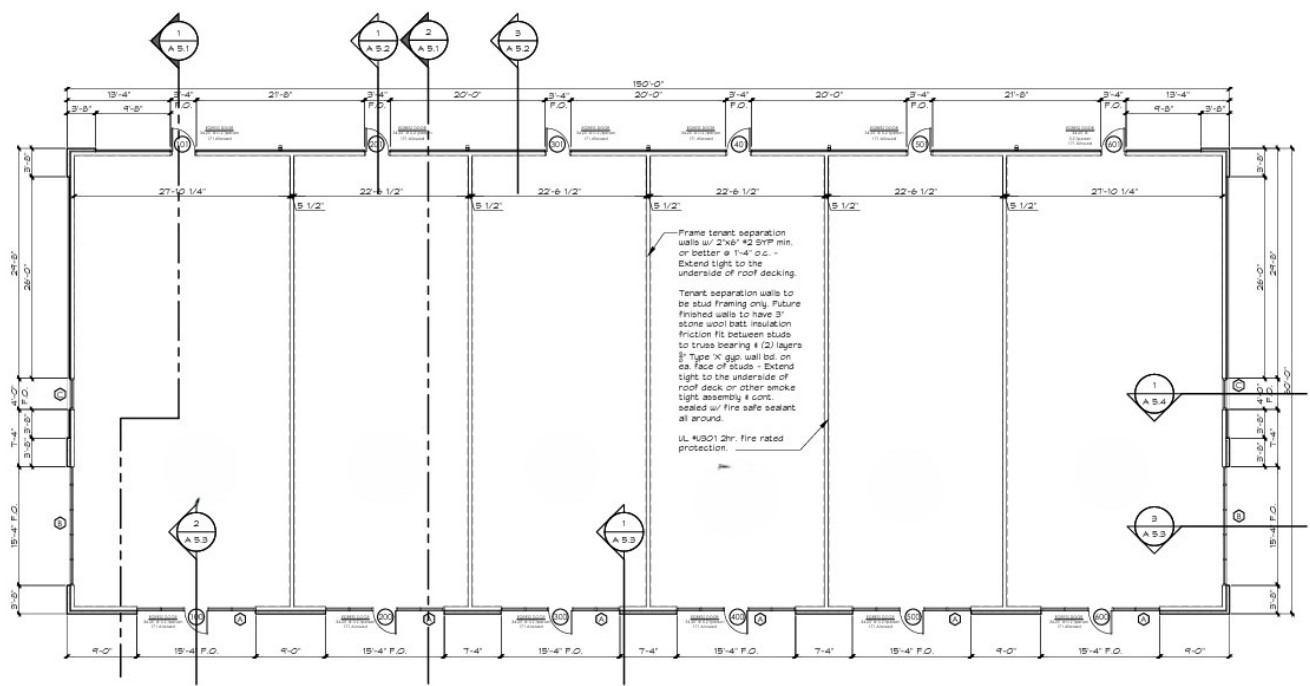
1 Floor Plan A-S.1
