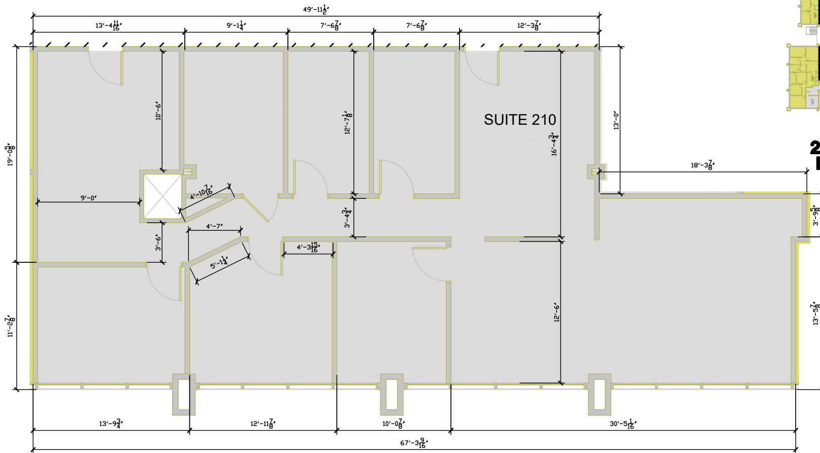
1 SUITE 210 TENANT PLAN SCALE: 3/16" = 1'-0"
