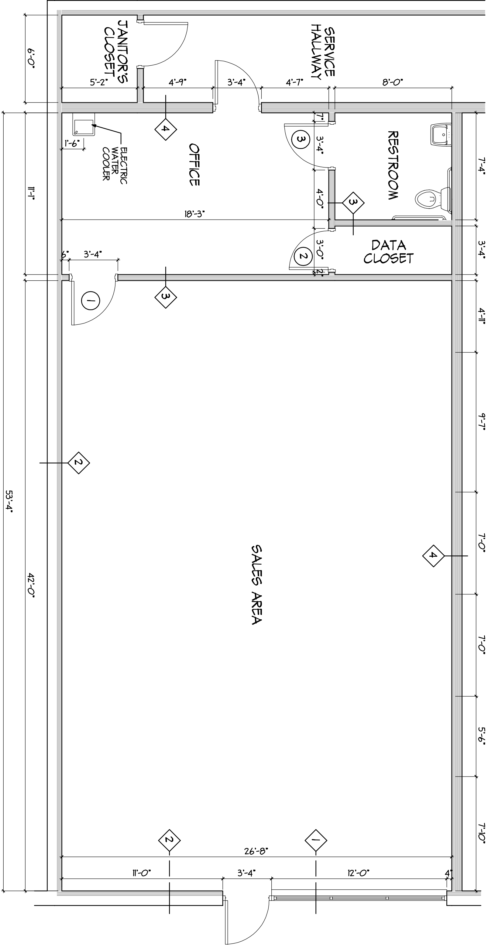
1 FLOOR PLAN A-1 SCALE: 1/4" = 1'-0"
