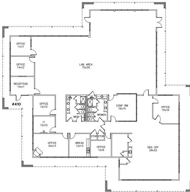
A FLOOR PLAN SCALE: 1/8" = 1'-0"
