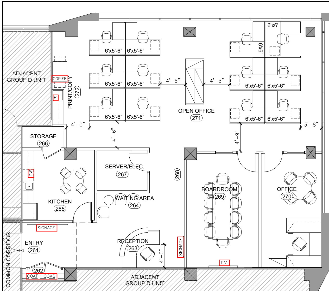
1 FURNITURE PLAN A3 SCALE: 1/8"=1'-0"
