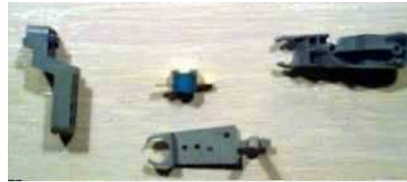
Soporte para termostatos de radiadores. Material PA 6.6 V-0
