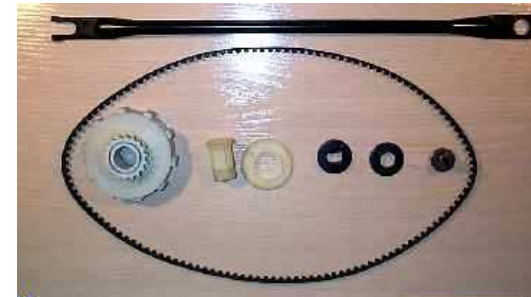
Movimiento sillón Citroën.
