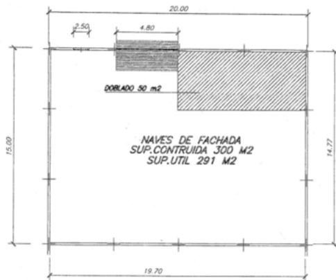
TIPO NAVE FACHADA A CALLE DE POLIGONO 3 UNIDADES
