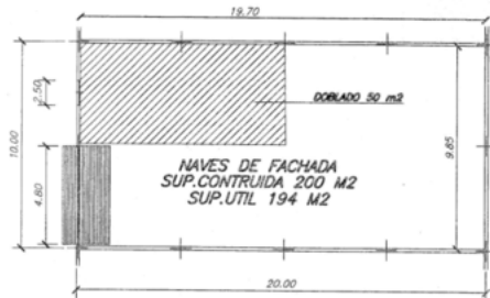
TIPO NAVE FACHADA A CALLE INTERIOR 13 UNIDADES
