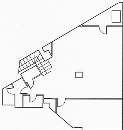
PLANTA SÓTANO
