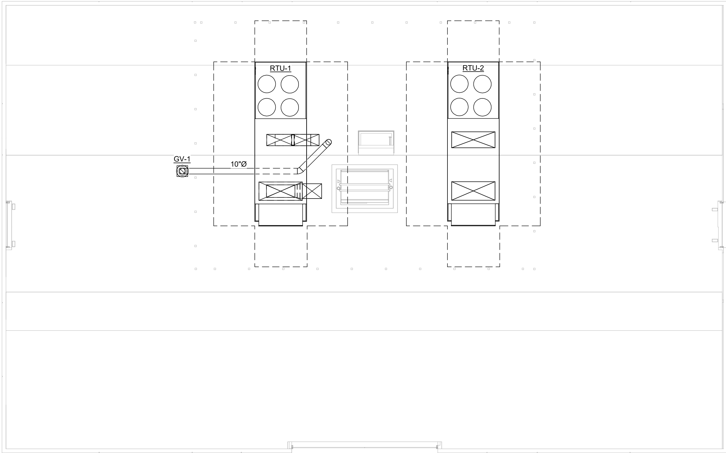
1 M-102 HVAC ROOF PLAN SCALE: 1/8" = 1'-0" N
