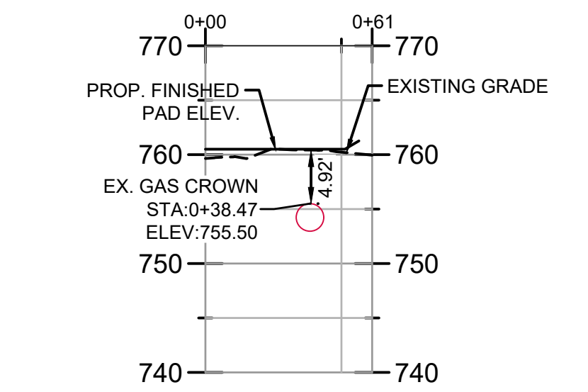
CROSS SECTION @ STA. 27+00 SCALE: N.T.S.
