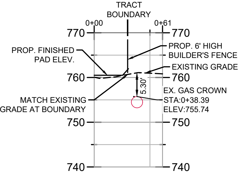
CROSS SECTION @ STA. 26+00 SCALE: N.T.S.
