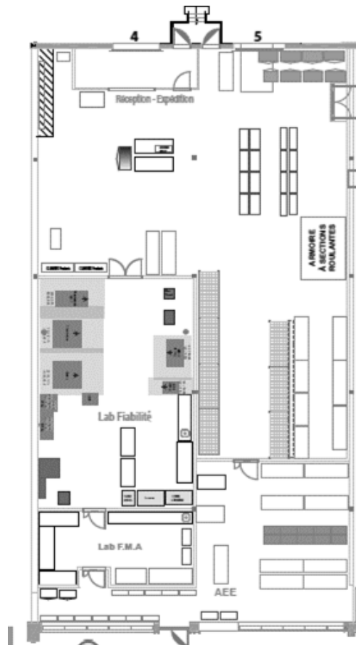
Plan d'étage (aménagé) Floor Plan (Built out)
