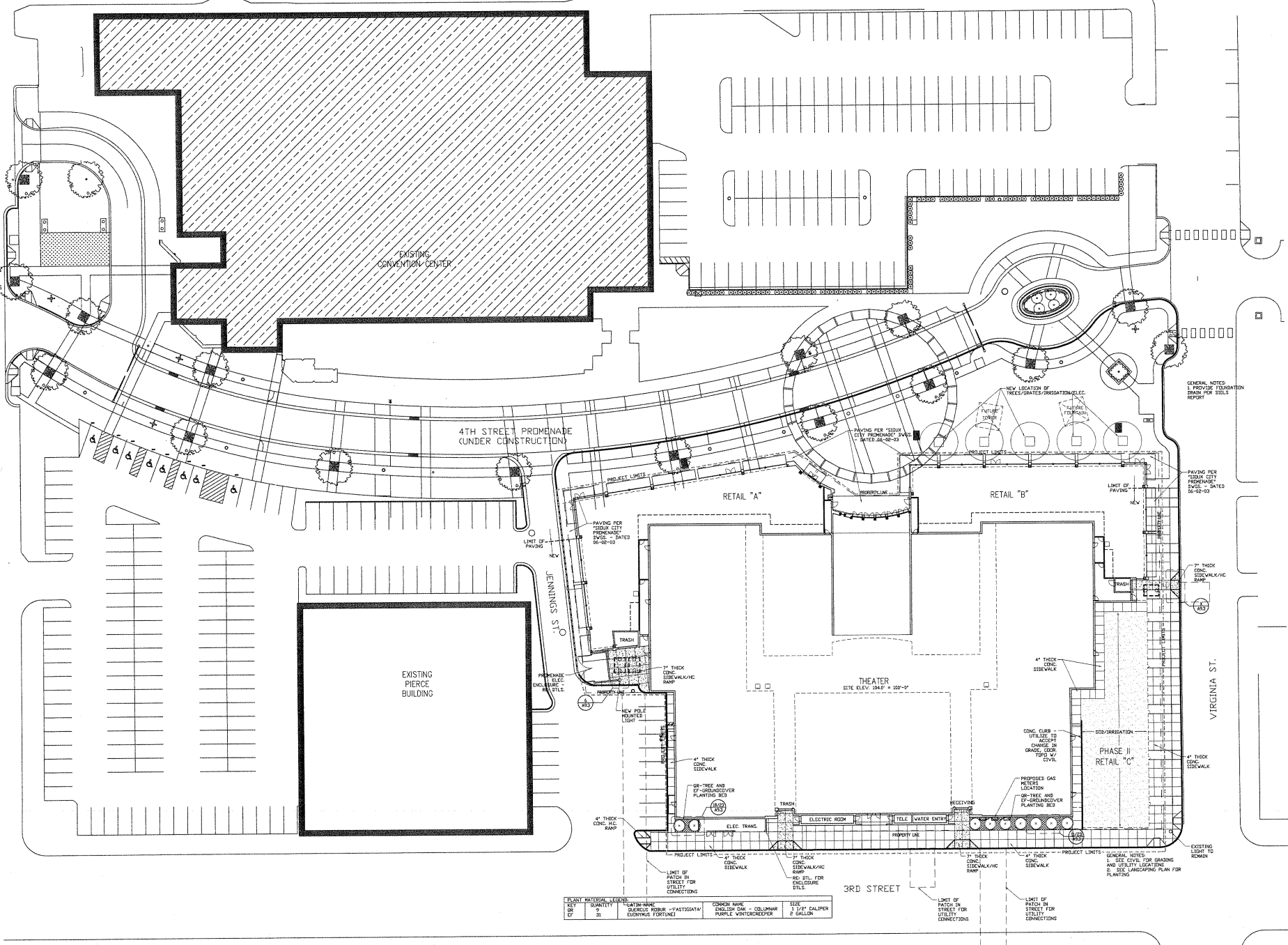
1 SITE PLAN SCALE: 1" = 20'
