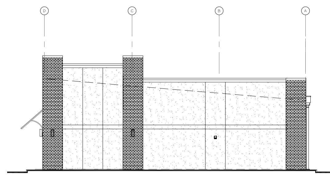
RIGHT ELEVATION BLDG 2 & 3
