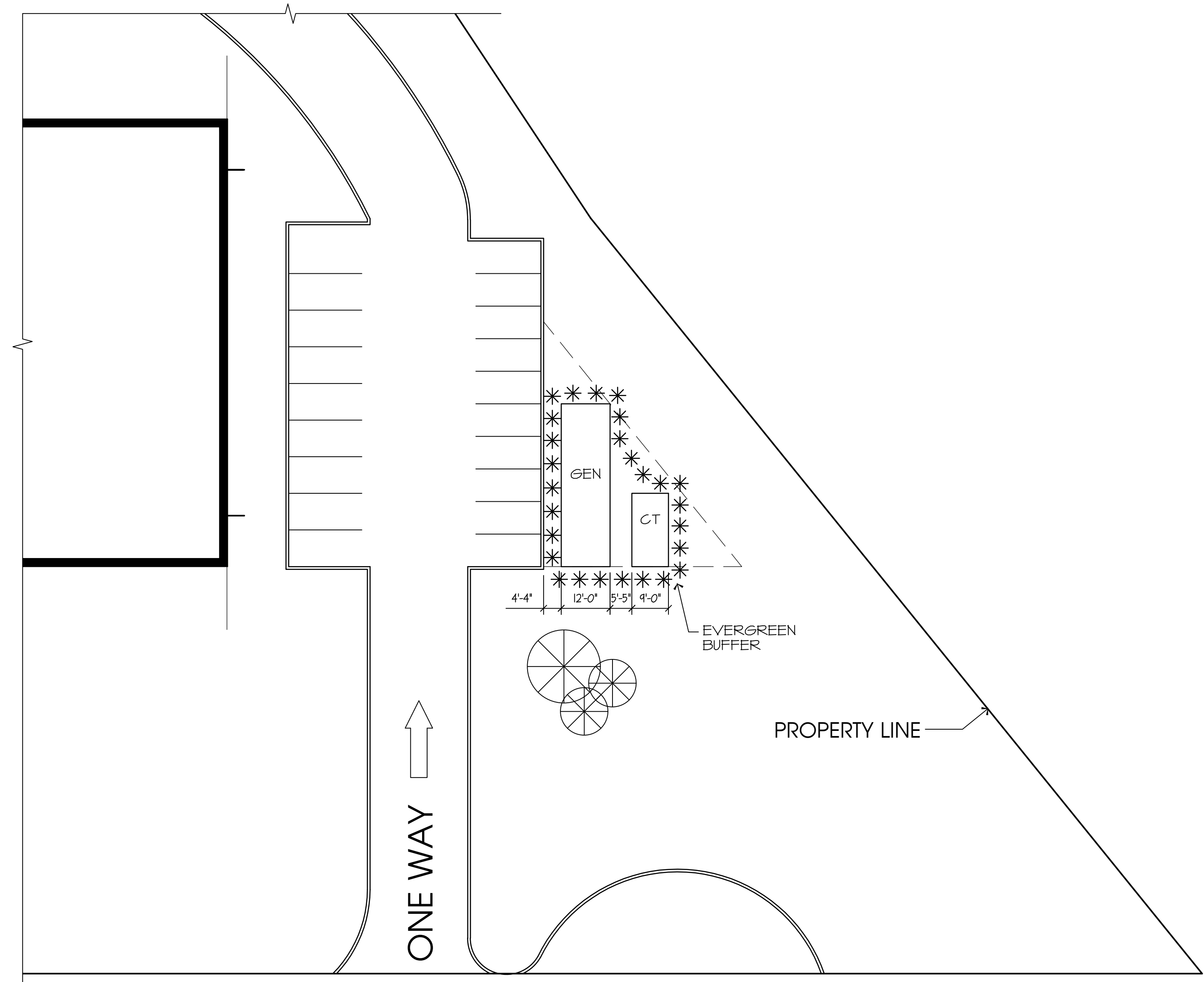
Plan scale: 1" = 20'-0"
