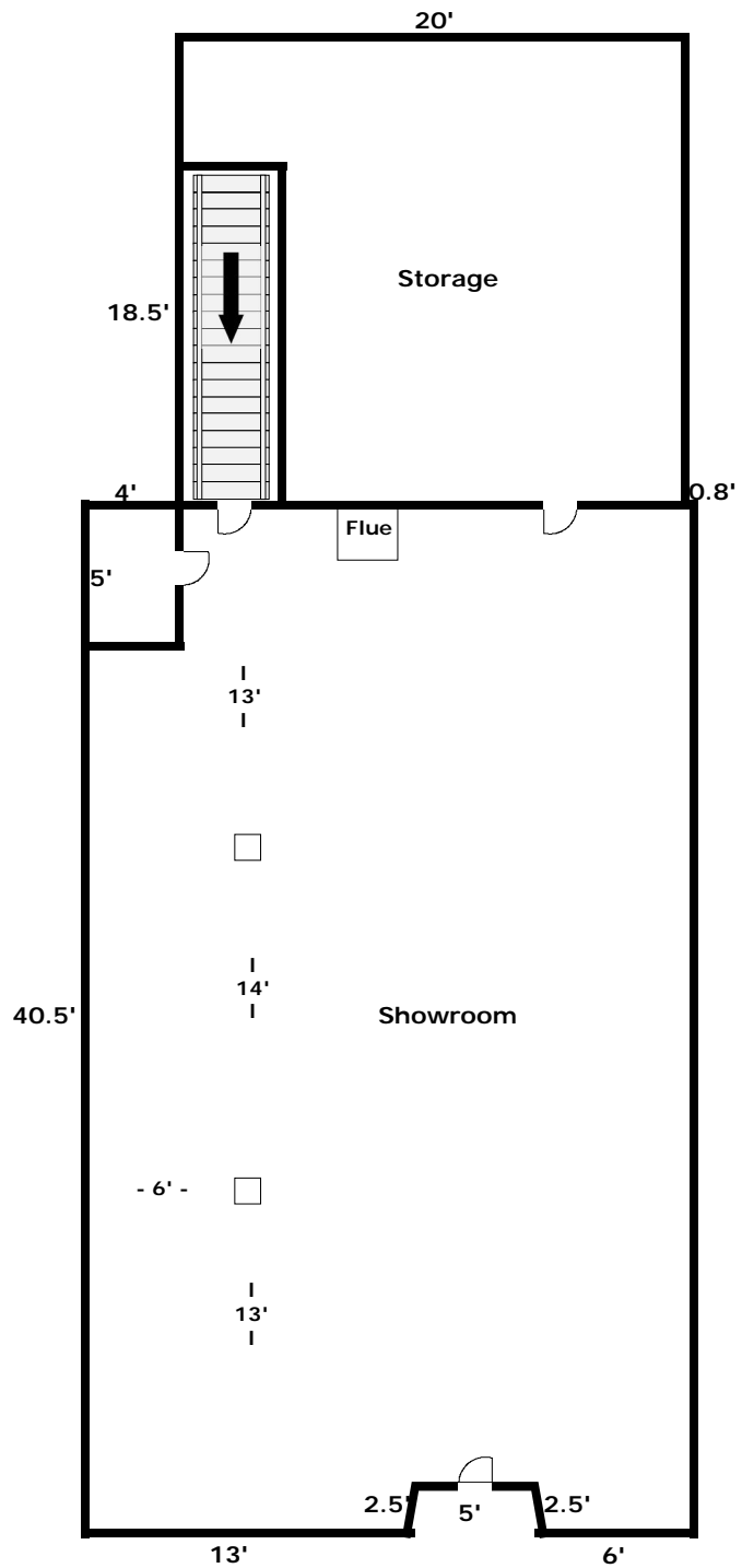
901 S. COLORADO, SALEM, VA FIRST FLOOR - 1,382+/- SF
