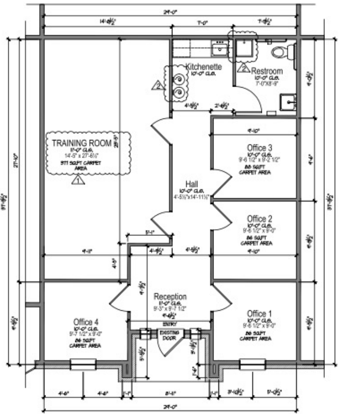
Dimensioned Floor Plan SCALE: 1/8"=1'-0" (VERT)
