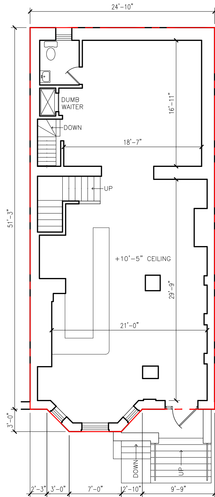
FIRST FLOOR / SCALE: 1/8" = 1'-0"
