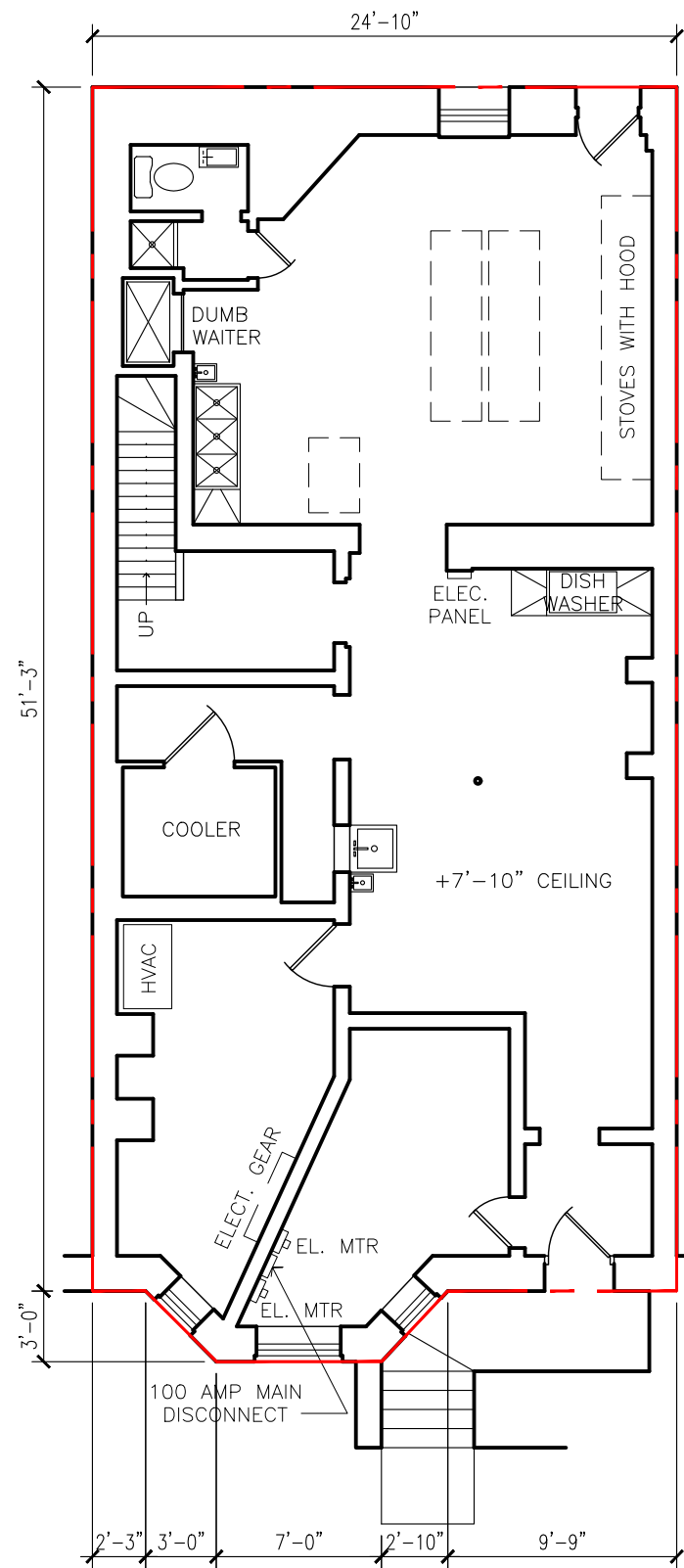
BASEMENT / SCALE: 1/8" = 1'-0"
