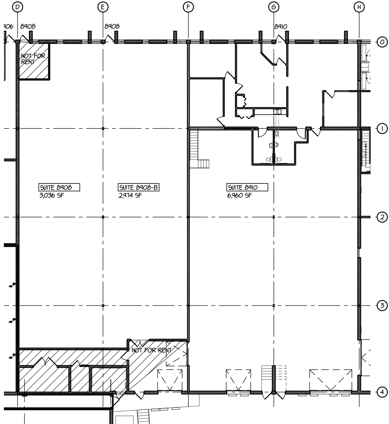
TENANT PLAN - SUITE 8908, 8908B & 8910 3/32" = 1'-0"
