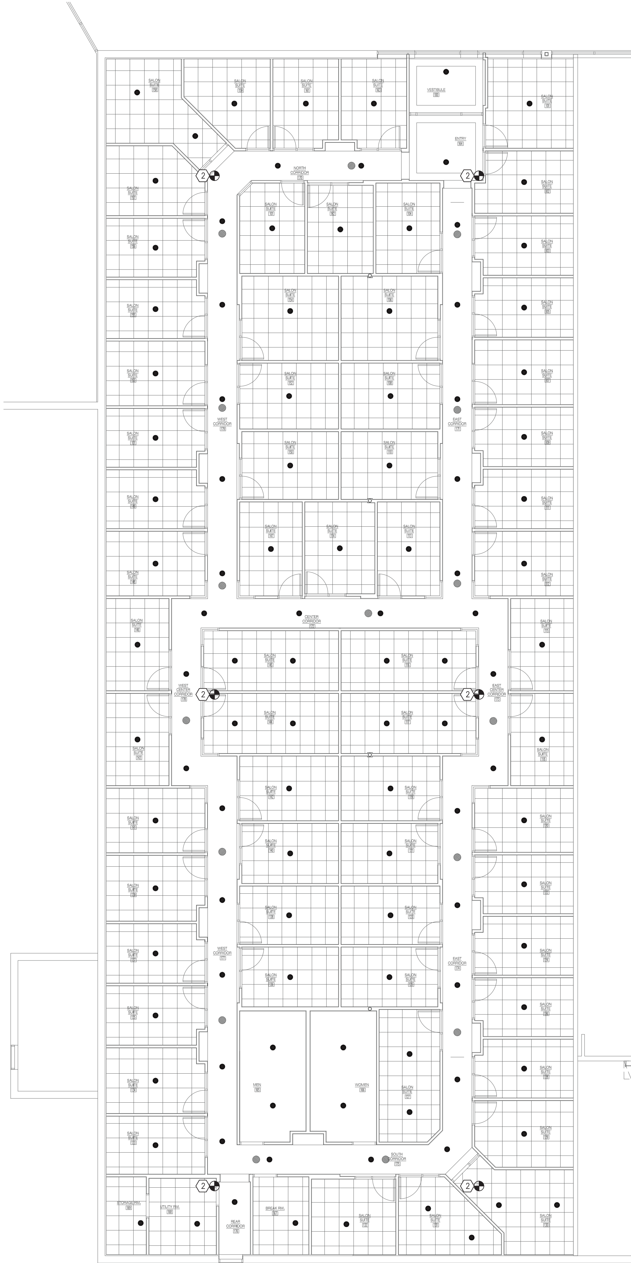
2 FIRE PROTECTION PLAN SCALE: 1/8" = 1'-0"
