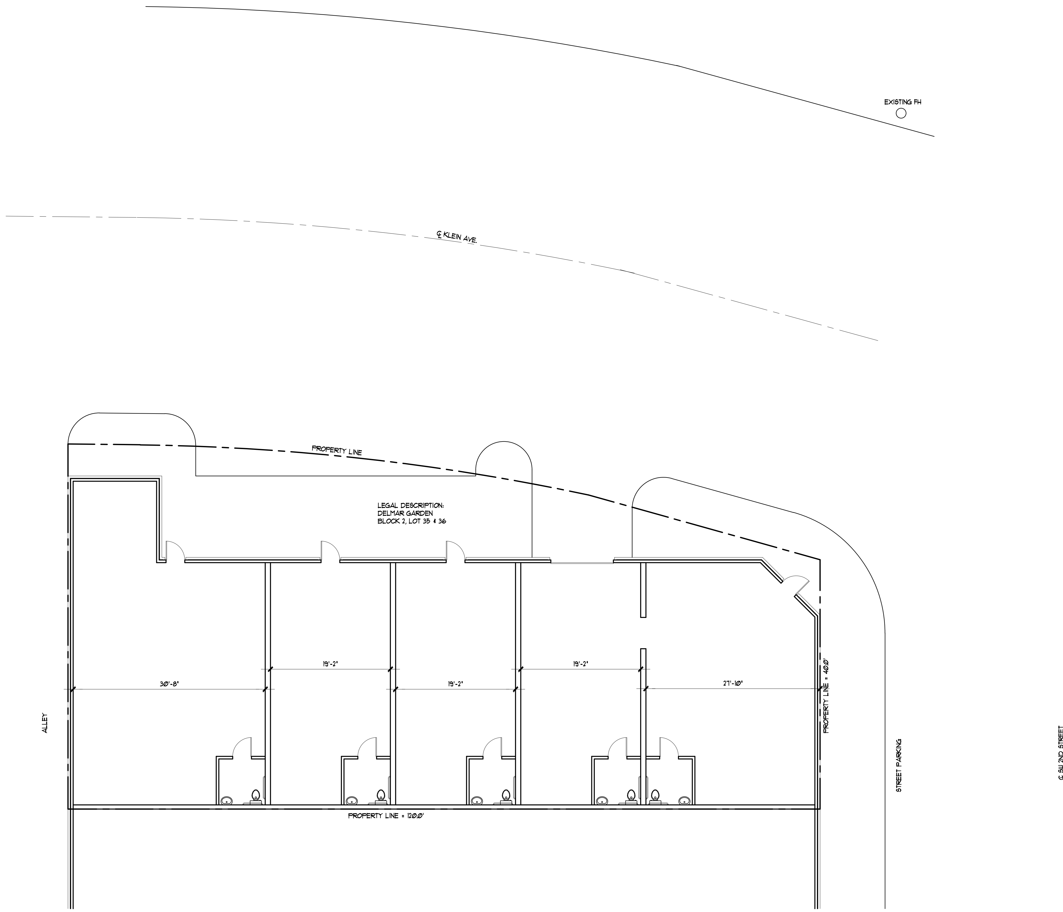
1 SITE PLAN A11 SCALE: 1/8" = 1'-0"
