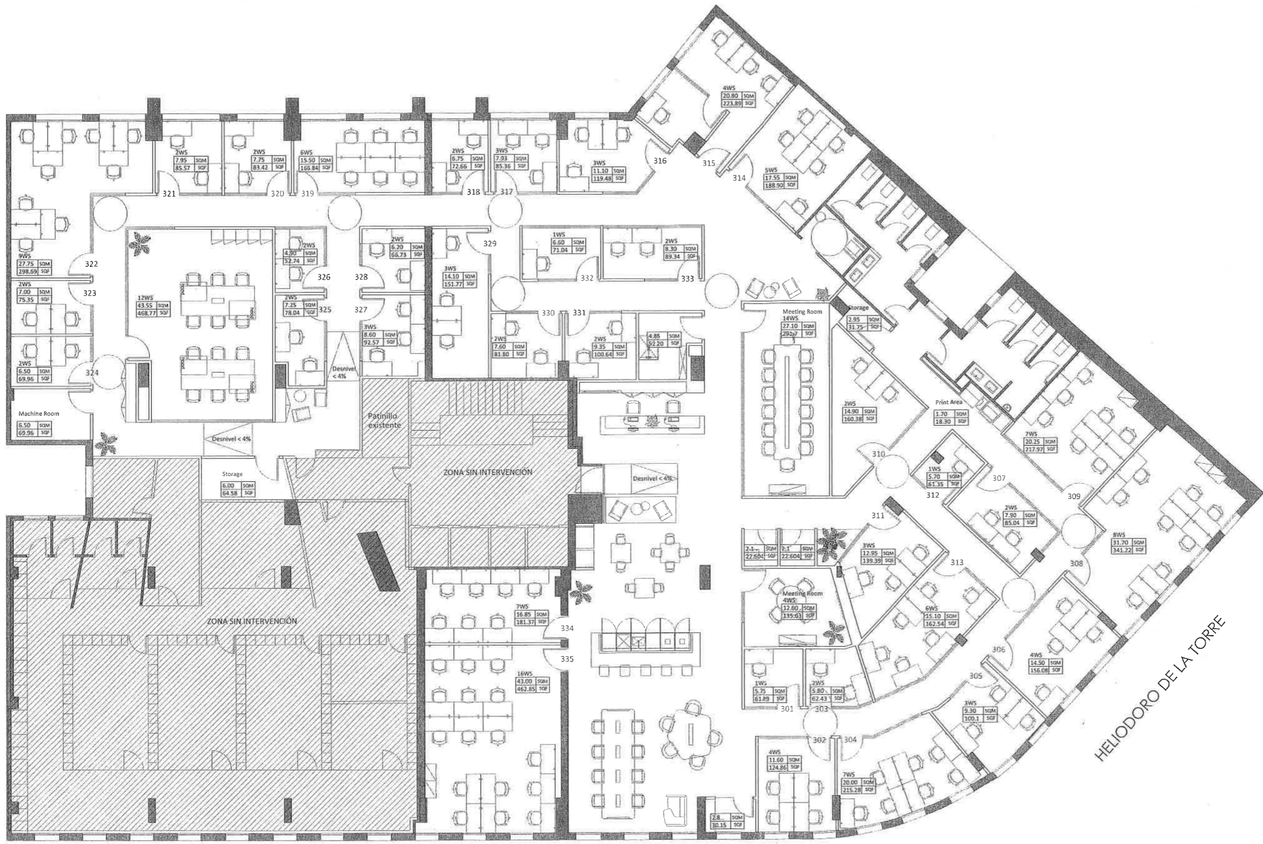
PLANTA TERCERA ESTADO REFORMADO
