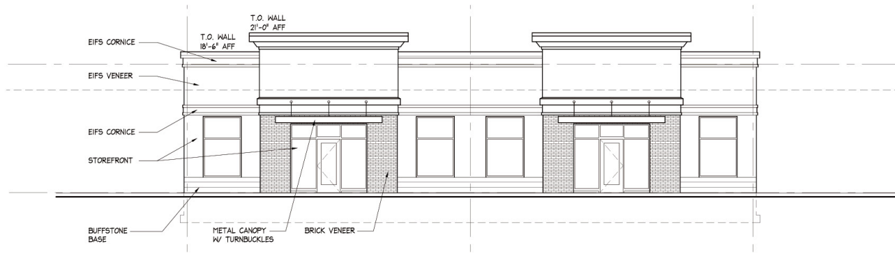
4 FRONT ELEVATION SCALE: 1/8" = 1'-0"
