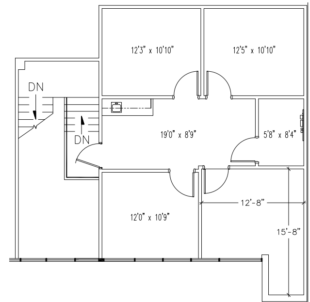
SUITE B (MEZZANINE) 828 SF
