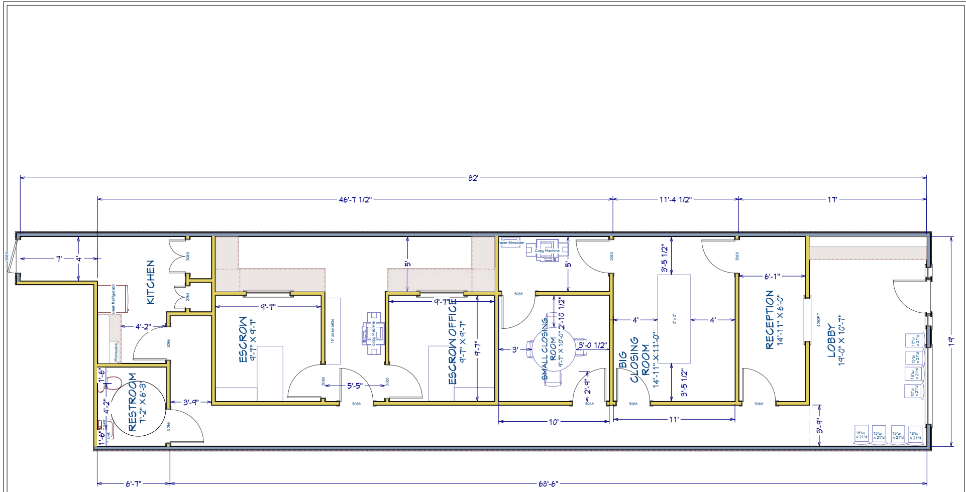
FLOOR PLAN SCALE: 3/8" = 1'-0"
