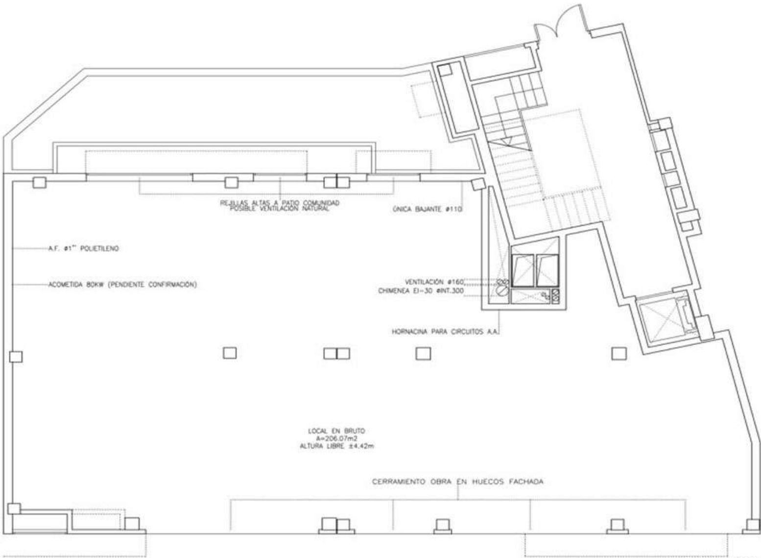
PLANTA LOCAL SUPERFICIE ÚTIL BRUTA LOCAL: ±206.10m 2
