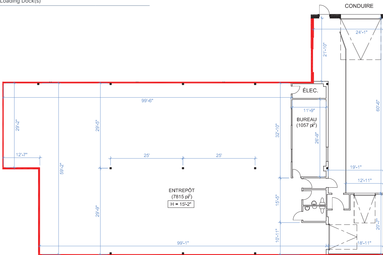
PLAN D'EMPLACEMENT
