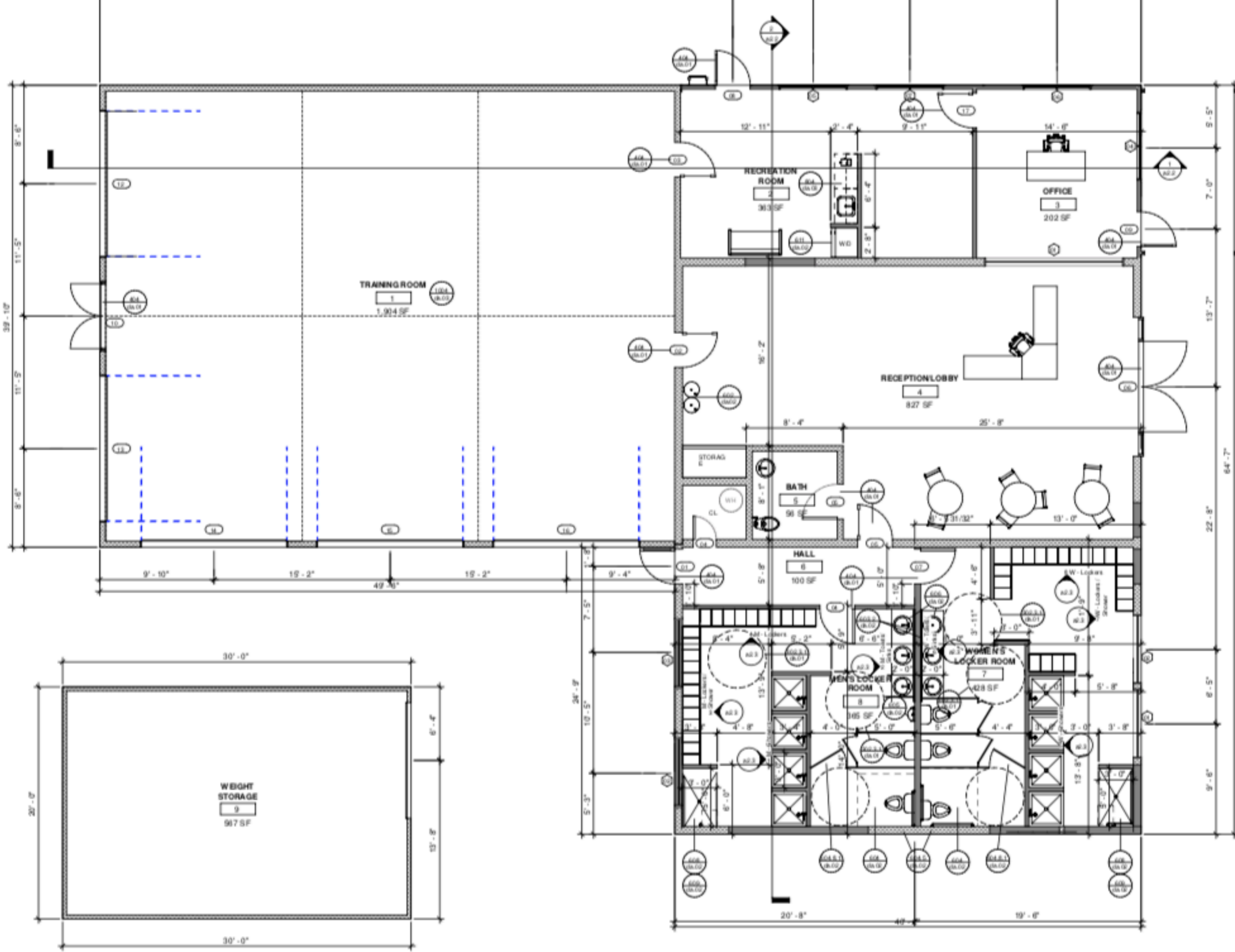
1 m/FFPLAN SCALE: 1/4" = 1'-0"
