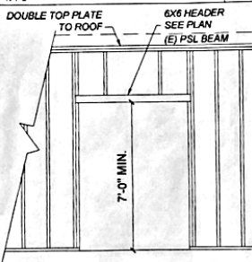
OPENING ELEVATION N.T.S.
