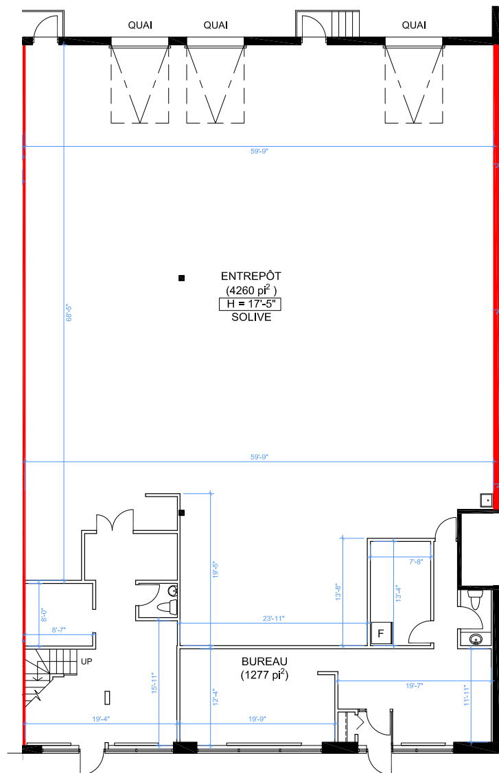
PLAN D'EMPLACEMENT
