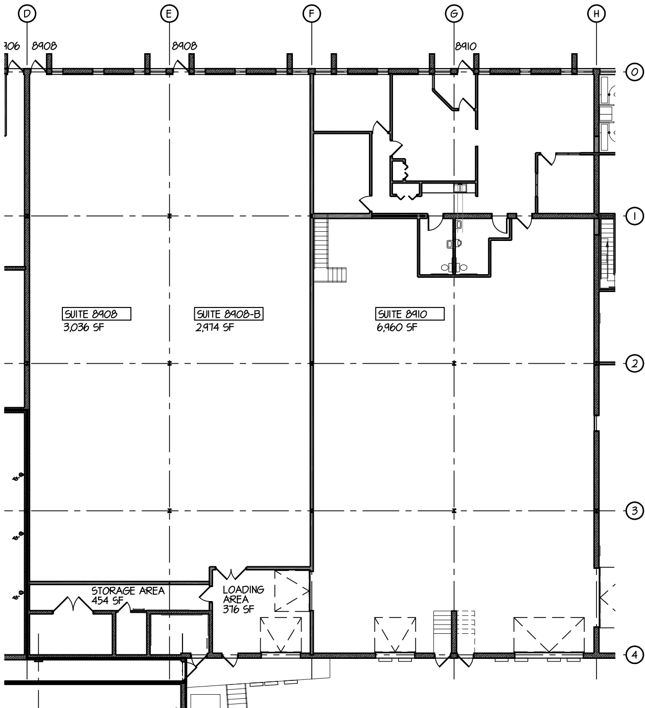
○ TENANT PLAN - SUITE 8908, 8908B & 8910 (13,800 S.F.) 3/32" = 1'-0"
