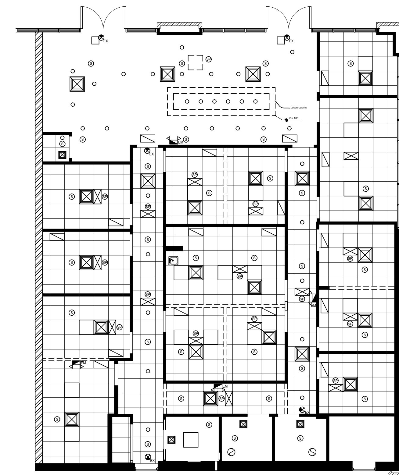
RCP LEGEND / SCALE: 1/8"=1'-0"
